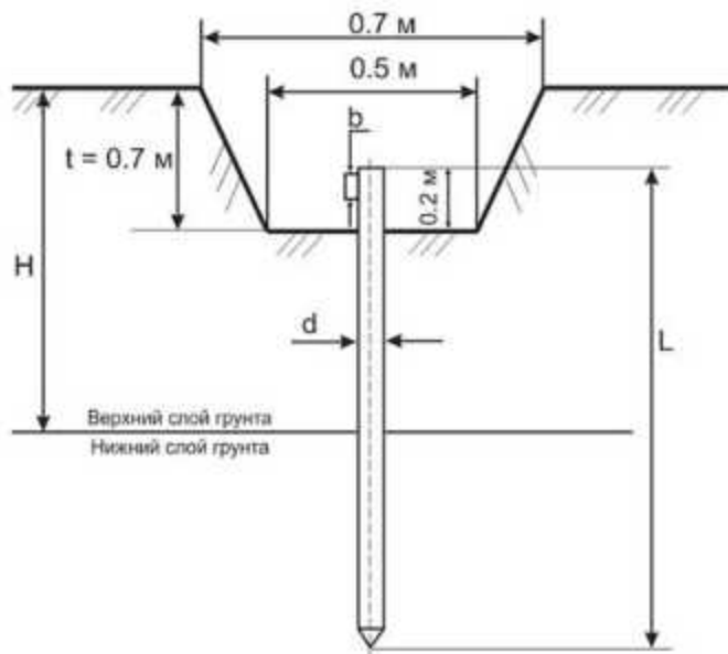
Рис. 3. Стержневой заземлитель
