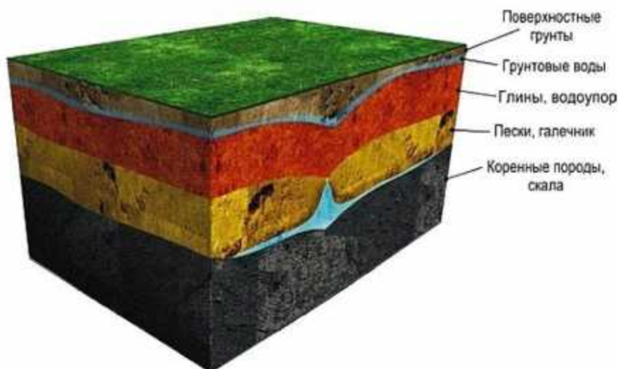
Рис. 1. Условный вид геологического строения грунта
