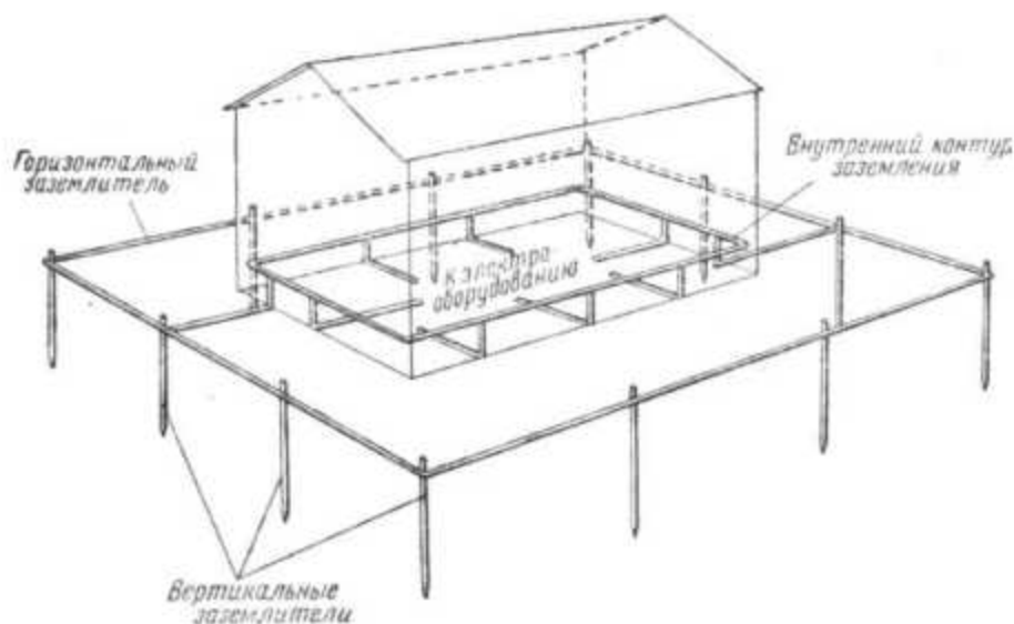
Рис. 4. Комбинированный заземлитель
